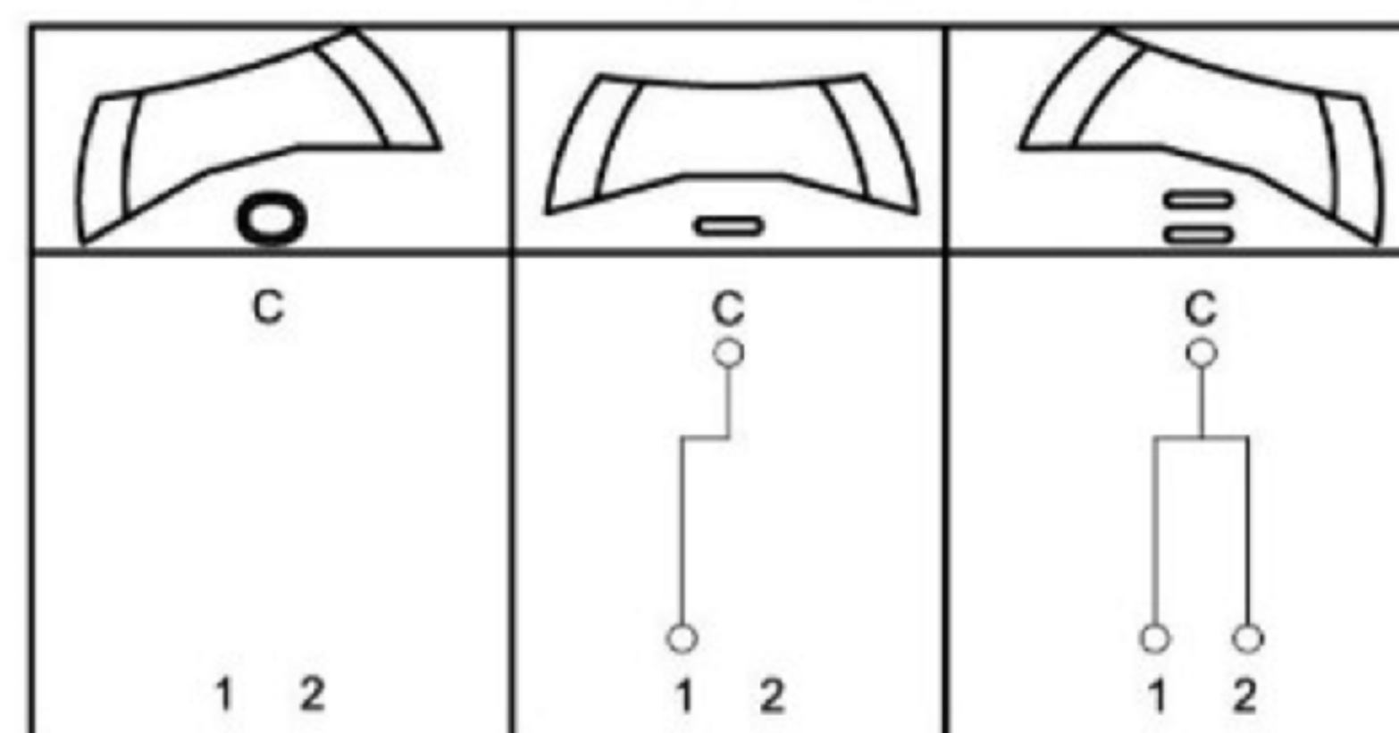
线路/ Circuit
