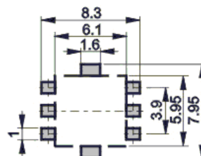
P.C.B.Land Pattern
