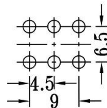
P.C.B LAYOUT
