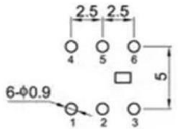
印制电路板 printed-circuit board
