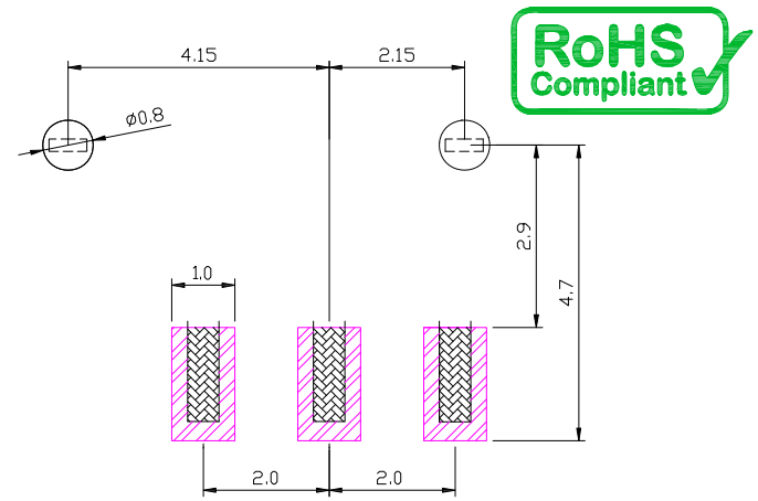
P.C.B LAND PATTERN
