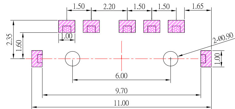
P.C.B LAND PATTERN
