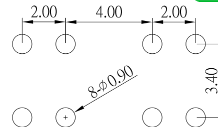
P.C.B LAND PATTERN
