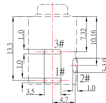
P.C.B LAYOUT
