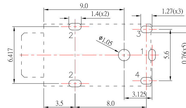
P.C.B LAYOUT
